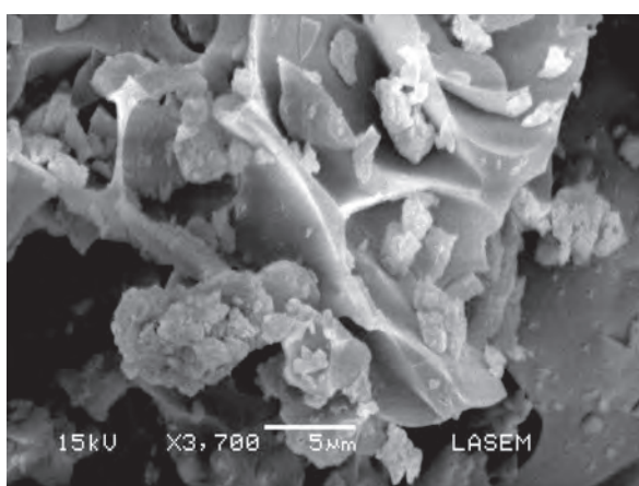
Figura 1: Vista al microscopio de una muestra de ceniza volcánica correspondiente a la erupción del Calbuco en el 2015.
