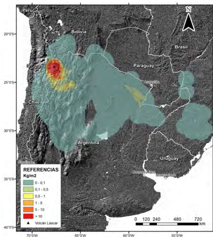
Figura 12. Dispersión de ceniza volcánica del Volcán Láscar correspondiente al evento de abril del 1993, simulada por el programa ATLAS. 39 horas después de iniciada la erupción.
