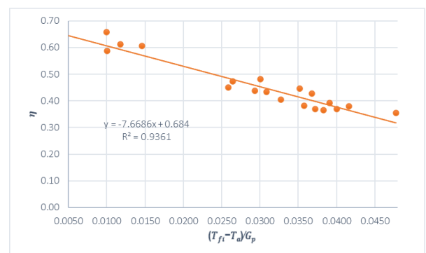
Fig. 20: Curva de eficiencia instantánea del colector cuña con malla porosa para el flujo másico de 0,025 Kg/s.
