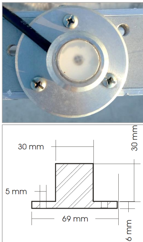
Fig. 1: Imagen del radiómetro fotovoltaico instalado del DES y dimensiones del instrumento.
