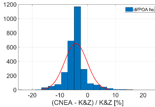
Fig. 3: Distribución de la diferencia porcentual de las integrales horarias entre las mediciones registradas por el dispositivo de referencia (K&Z) y el radiómetro del DES (CNEA).
