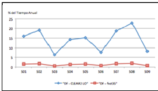
Fig. 9: porcentaje de tiempo anual en función del DF establecido por la normativa, para los distintos puntos medidos.
