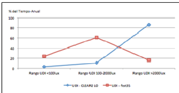
Fig. 10: porcentaje del tiempo anual en función de los rangos del parámetro UDI, para los distintos puntos medidos.
