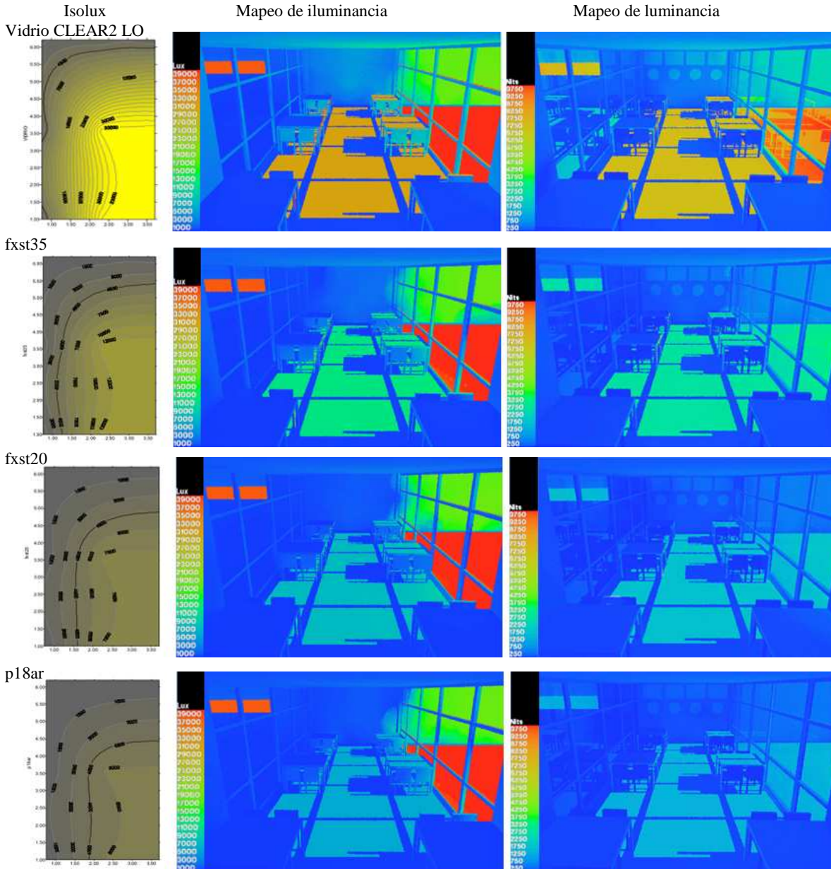
Fig. 8: curvas de isolux, mapeos de iluminancia y mapeos de luminancia.
