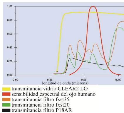
Fig. 17: curvas de transmitancias de los elementos transparentes y curva de sensibilidad espectral del ojo humano.
