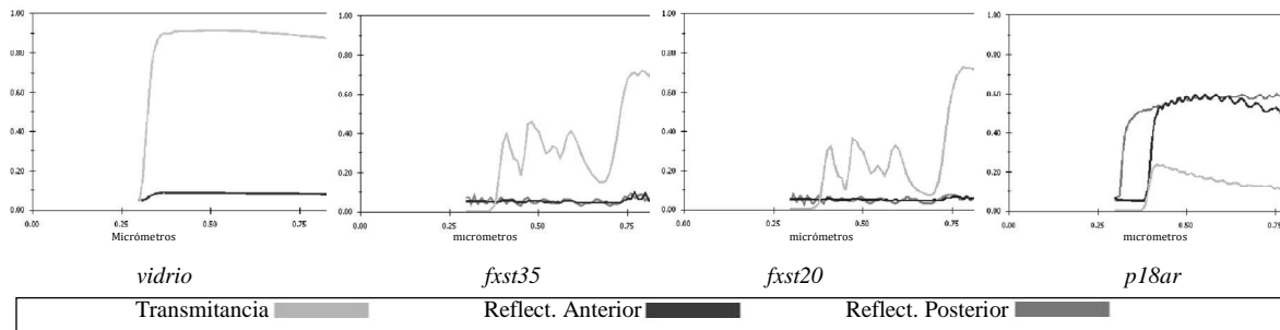
Fig. 4: curvas de transmitancia y reflectancia del vidrio y los filtros seleccionados. Optic5.
