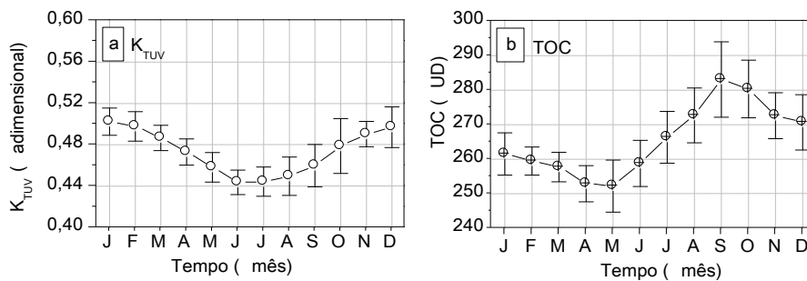
Fig. 8: Médias mensais interanuais da K_{TUV} em condições de céu claro (a) e da coluna total de ozônio TOC (b).
