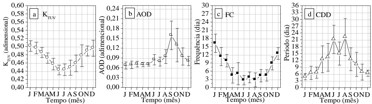
Fig. 4: Médias mensais interanuais dos valores diários de K_{TUV} em condições de céu claro (a), profundidade de ótica de aerossóis (b), frequência mensal de dias com chuva (c), período máximo de dias secos (d).
