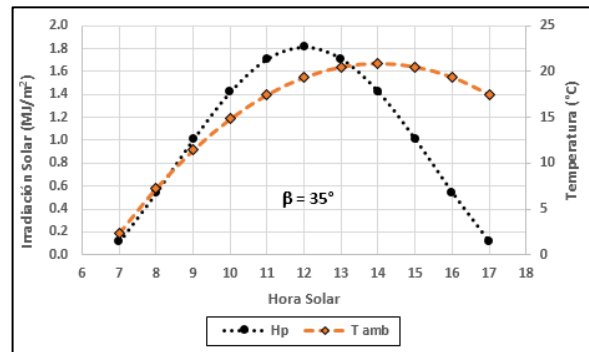
Fig. 2: Irradiación solar global horaria sobre el plano del colector y temperatura ambiente en el mes de julio.
