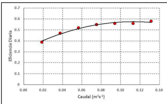
Fig. 4: Eficiencia diaria en función del caudal circulante.
