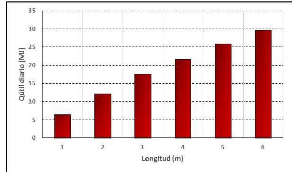
Fig. 9: Calor útil diario generado en función de la longitud del colector.
