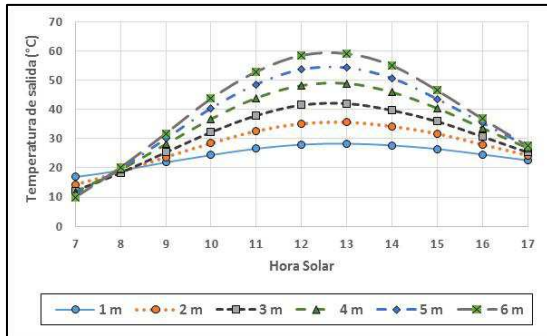
Fig. 7: Evolución temporal de la temperatura de salida del aire parametrizada con la longitud del colector.
