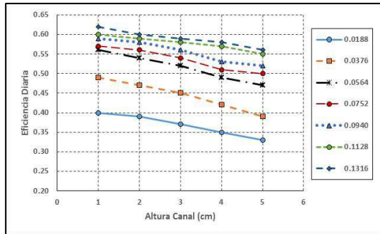
Fig. 11: Eficiencia diaria en función de la altura del canal de flujo y del caudal circulado.
