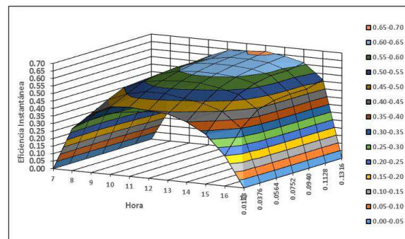
Fig. 6: Evolución horaria de la eficiencia térmica instantánea parametrizada con el caudal de circulación.
