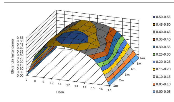
Fig. 10: Eficiencia térmica instantánea parametrizada con la longitud del colector.
