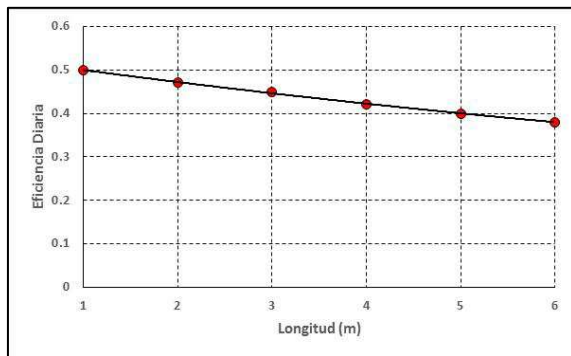
Fig. 8: Eficiencia diaria en función de la longitud.
