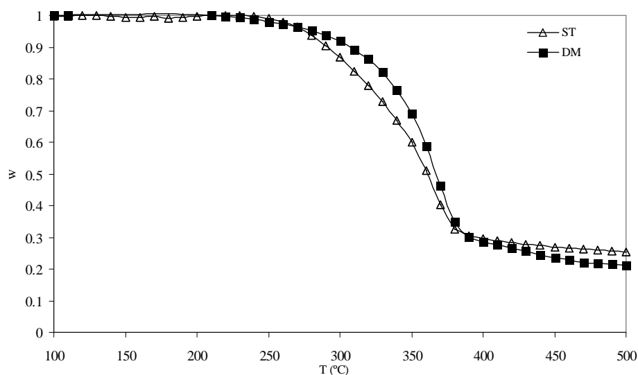
Figura 1: Curvas termogravimétricas para la pirólisis del aserrín sin tratar (ST) y demineralizado (DM).
