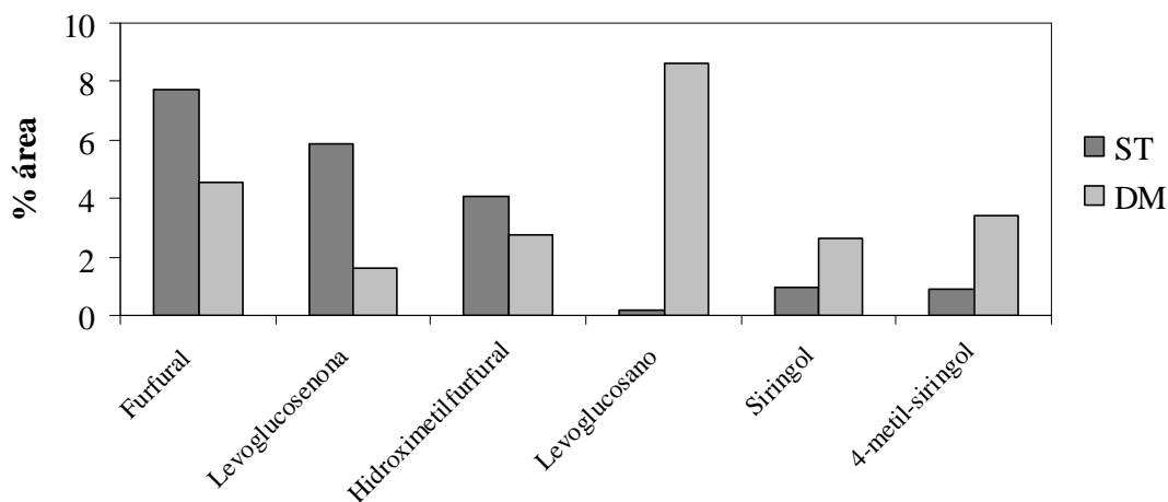
Figura 6: Productos característicos de la pirólisis (en % de área relativa) del aserrín sin tratar (ST) y demineralizado (DM)
