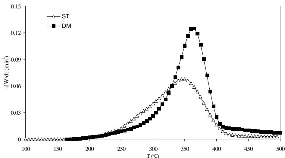
Figura 2: Efecto de la temperatura sobre las velocidades de degradación térmica del aserrín sin tratar (ST) y demineralizado (DM)
