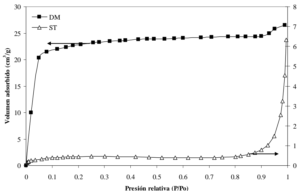
Figura 4: Isotermas de adsorción de N_2 (-196°C) para los bio-chars resultantes de la pirólisis del aserrín prístino (ST) y demineralizado (DM)
