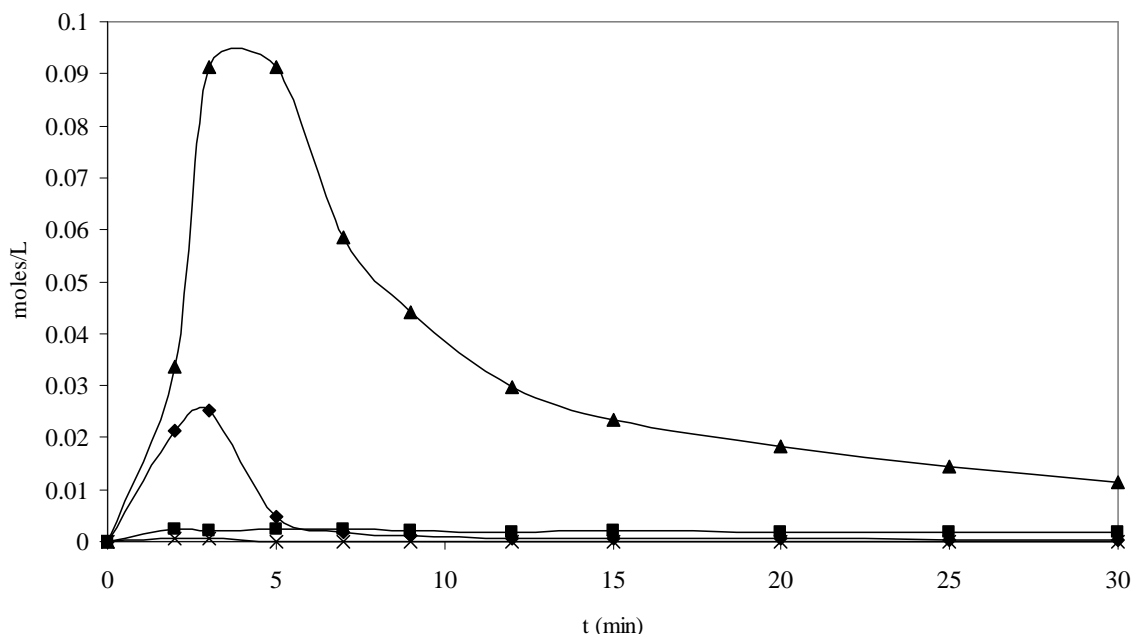
Figura 7: Evolución temporal de la concentración de las principales especies gaseosas producidas en la pirólisis del aserrín sin tratar. \blacktriangle : dióxido de carbono; \blacklozenge : monóxido de carbono; \blacksquare : metano; \times : hidrógeno.
