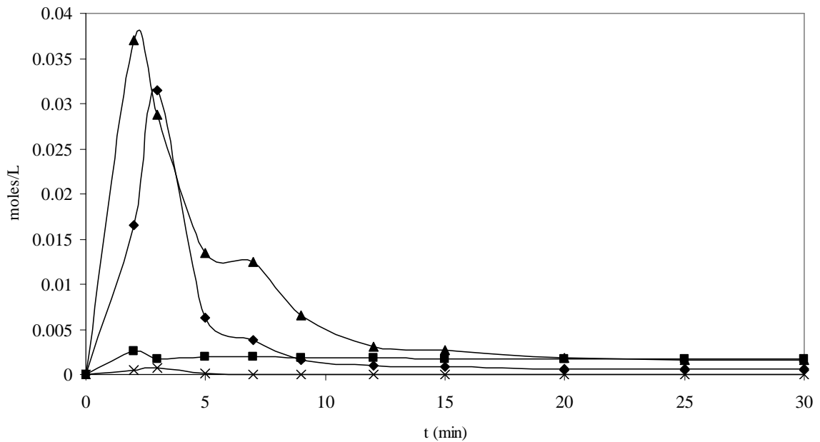
Figura 8: Evolución temporal de la concentración de las principales especies gaseosas producidas en la pirólisis del aserrín demineralizado. ▲ : dióxido de carbono; ◆ : monóxido de carbono; ■ : metano; × : hidrógeno.
