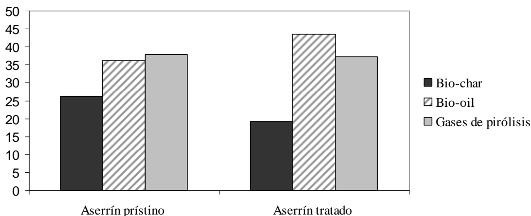
Figura 3: Efecto de la demineralización del aserrín de Cina-cina sobre los rendimientos de los tres tipos de productos de pirólisis.
