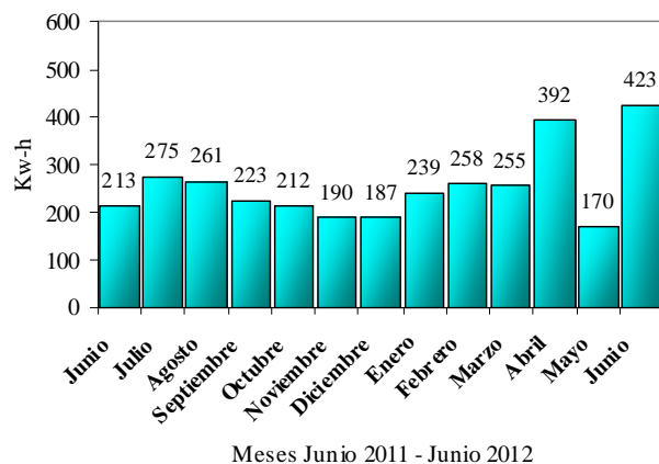
Figura 19: Consumo de energía eléctrica durante el año de medición
