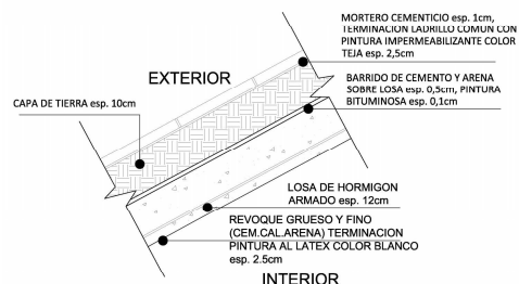
Figura 6: Corte del techo
