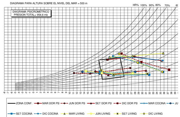
Figura 18: Diagrama psicrométrico planta baja Septiembre 2011 – Junio 2012
