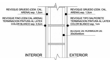
Figura 5: Corte de un muro de la casa
