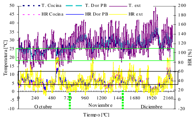
Figura 11: Comportamiento higrotérmico de la planta baja
