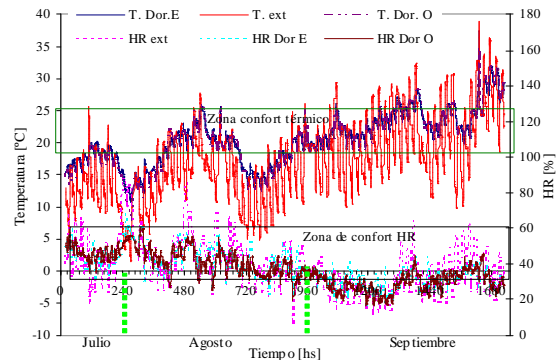
Figura 10: Comportamiento térmico de los dormitorios de la planta alta Julio Septiembre 2011
