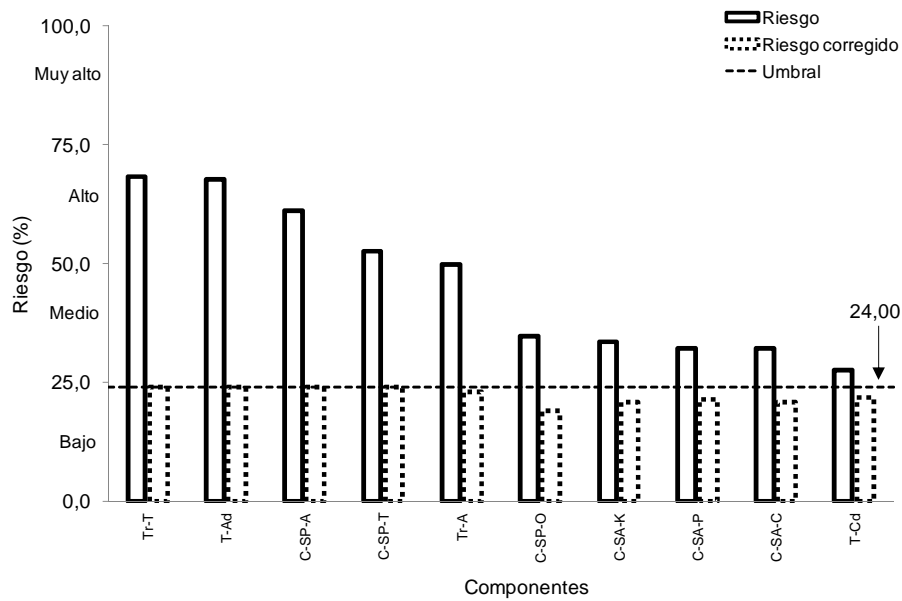
Figura 6. Riesgo actual y corregido para todos los componentes del sistema Finca las Costas. Código de procesos: C=Captación; T=Transporte; Tr=Tratamiento. Código de sub-procesos: SP=Superficial; SA=Subálvea; Ad=Aducción; Cd=Conducción. Código de componentes: A=Astilleros; T=La Toma; O=La Olla; K=Kilómetro Cero; P=Peñalba.
