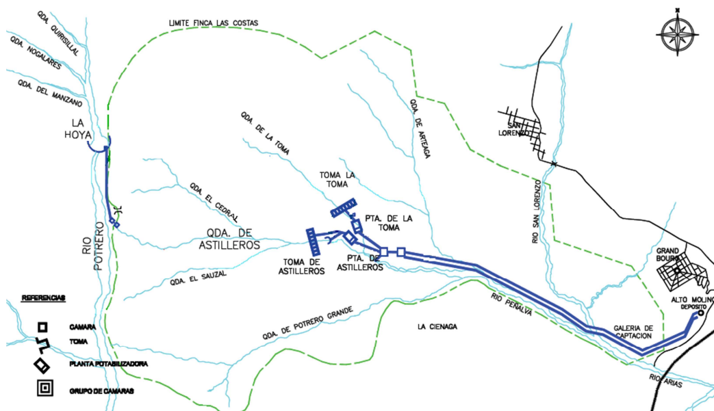
Figura 1. Esquema del sistema de abastecimiento de agua Finca Las Costas (Fuente: CoSAySa).
