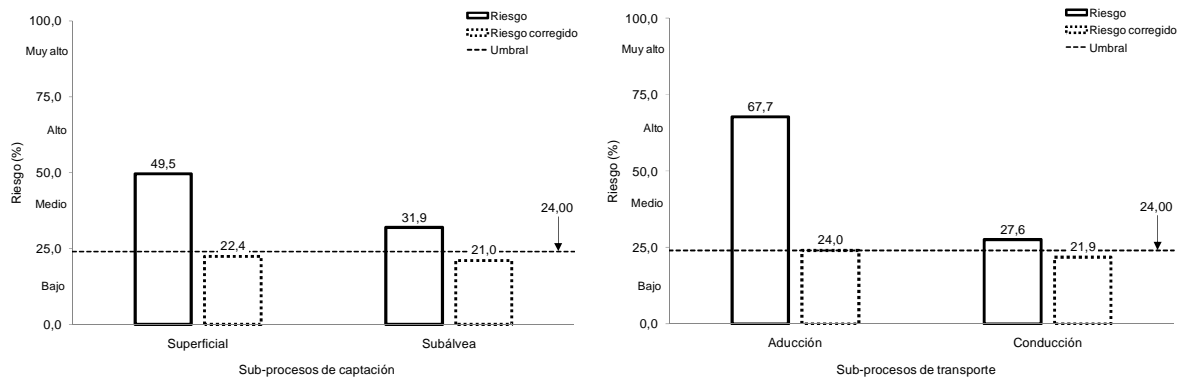
Figura 5. Riesgo actual y corregido de los sub-procesos de Captación (izquierda) y Transporte (derecha).
