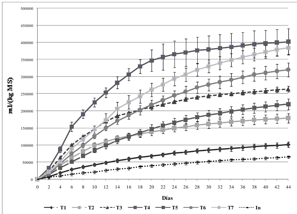
Figura 2: Producción de Biogás acumulada (ml/(kg MS)) en función del tiempo en días en los distintos tratamientos.
