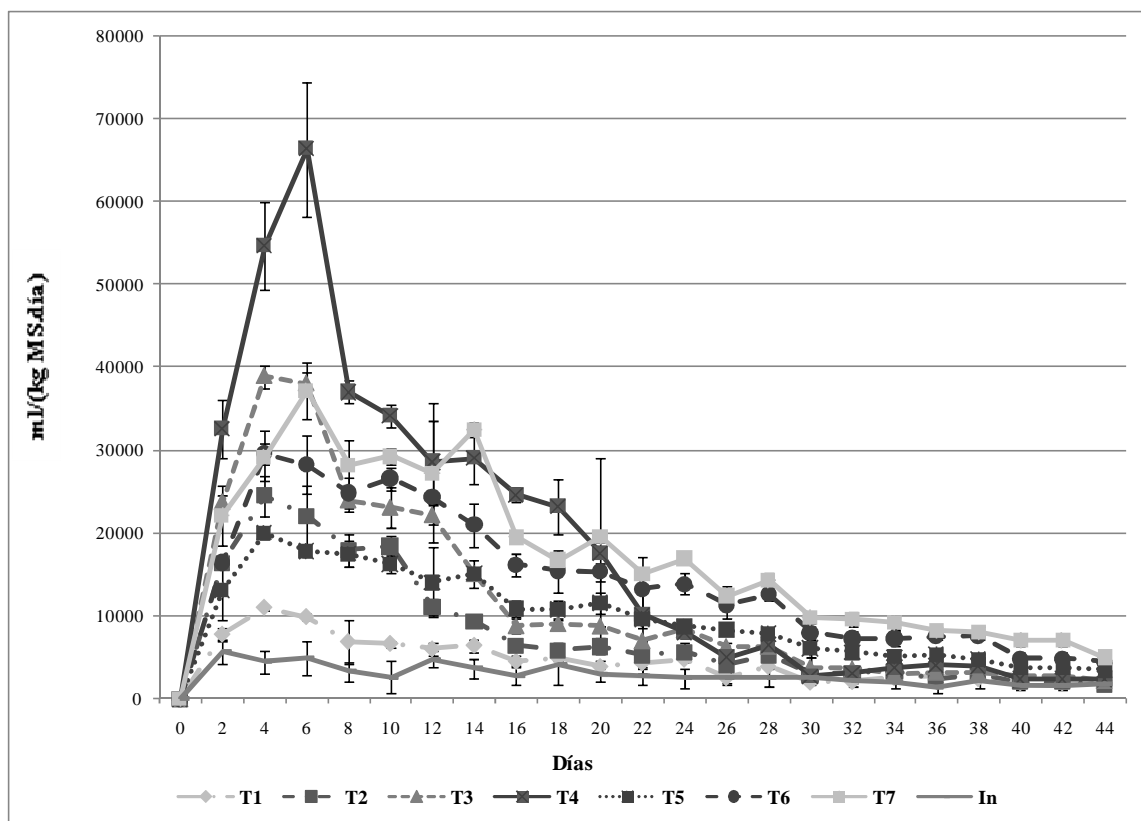
Figura 3: Producción diaria de Biogás (ml/(kg MS día)).
