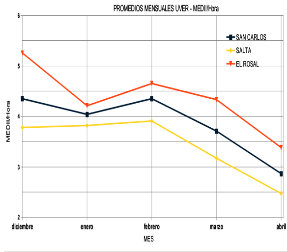
Fig 10: Distribución promedio mensual diaria de irradiación UV eritémica ( MED_{II}/hr ) en tres sitios de altura de la provincia de Salta
