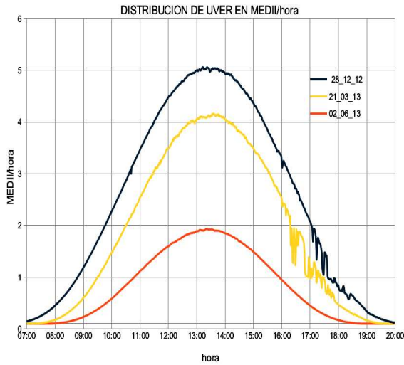
Fig 9: Distribución de irradiación UV eritémica ( MED_{II}/hr ) en Salta (Capital) para tres días claros a lo largo del período de medición.
