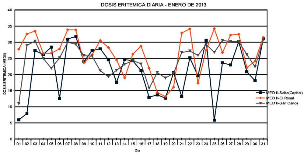
Fig 5: Dosis eritemica diaria en el mes de Enero del 2013 en tres sitios de altura de Salta.
