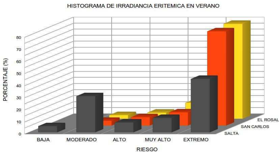
Figura 11: Histograma de ocurrencia de irradiación UV eritémica clasificados por riesgo solar durante el verano en Salta (Capital), San Carlos y El Rosal.
