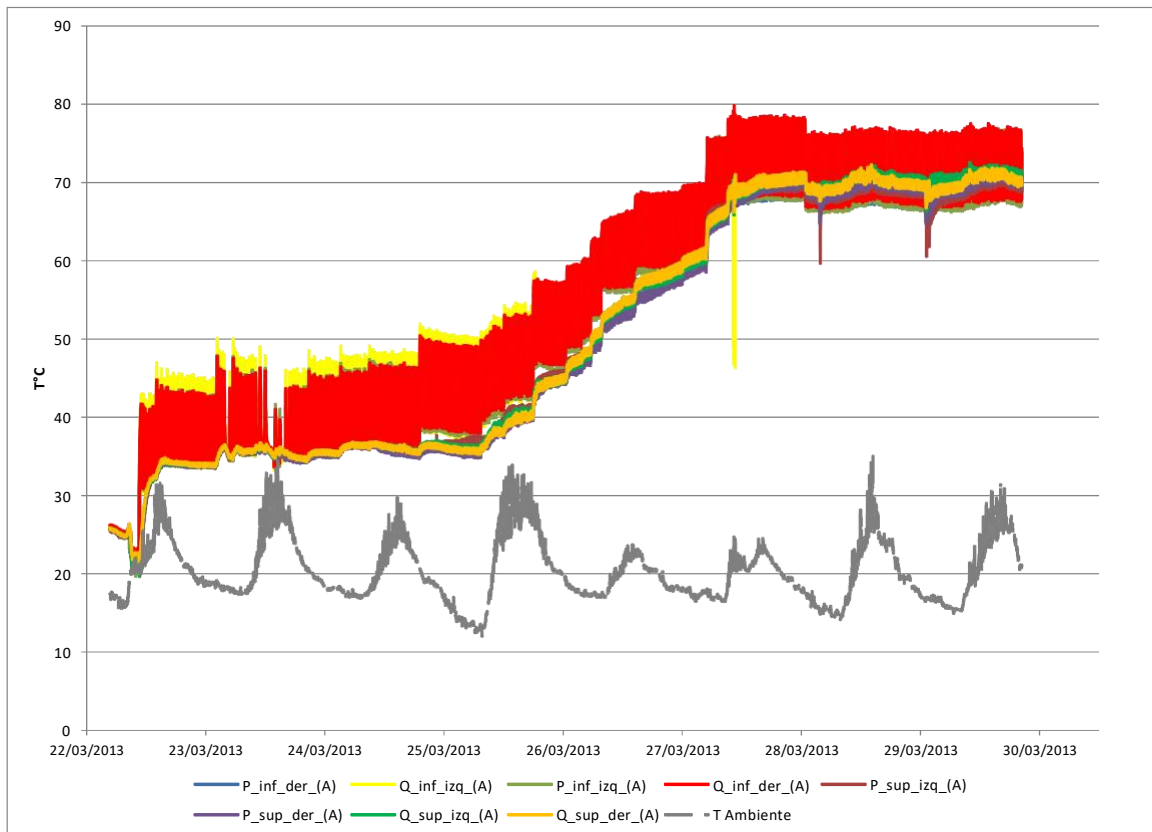
Figura 2: Datos de temperatura registrados en la estufa con Arena y Ripio (A)
