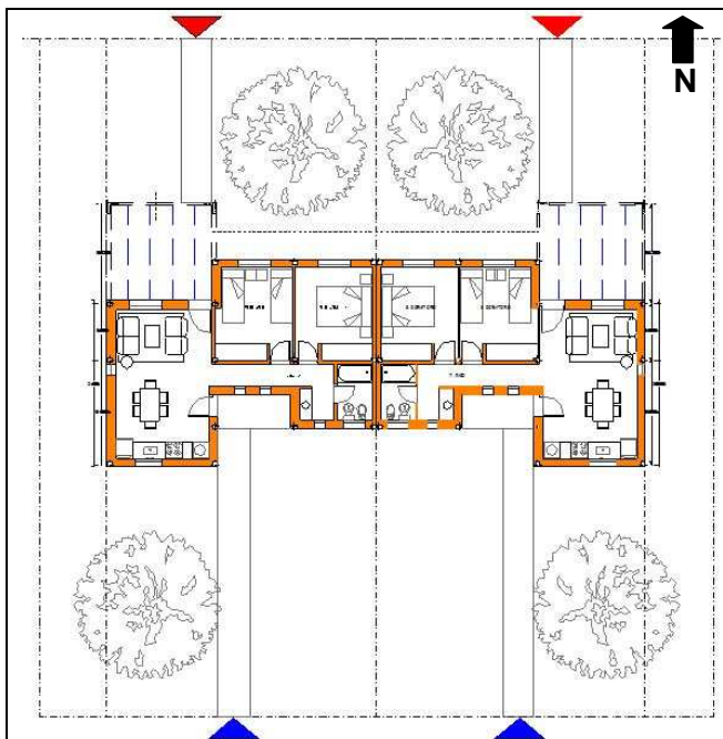
Figura 7: Plantas de la vivienda con acceso Norte o Sur
