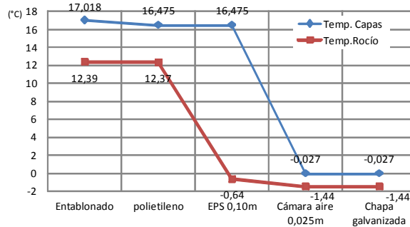
Figura 11: Verificación de riesgo de condensación de cubiertas de las viviendas para las diferentes categorías de análisis.
