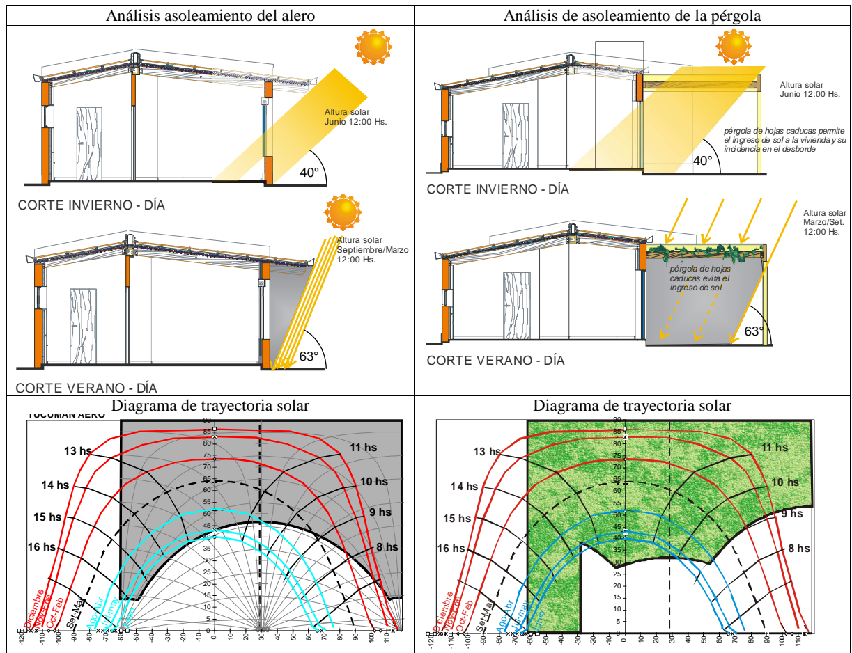
Figura 14: Evaluación de comportamiento de las protecciones solares de la fachada norte de las viviendas categoría 3 y 4.
