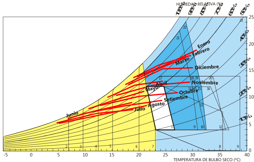
Figura 3: Diagrama psicrométrico con valores de temperatura y humedad de la localidad de análisis.
