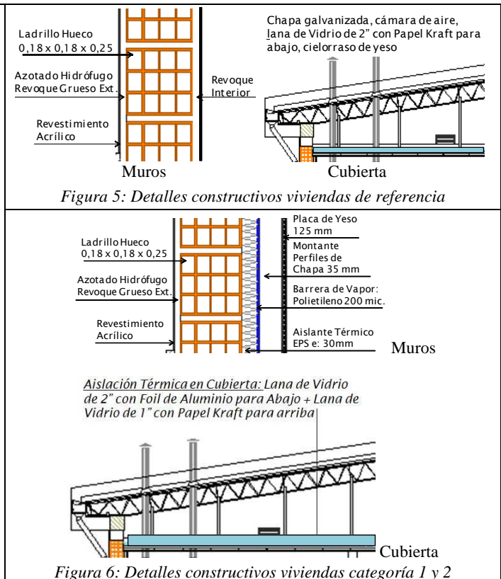
Figura 4: Vivienda de referencia y categoría 1 y 2
