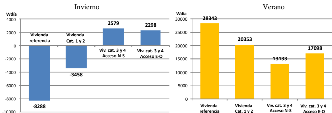
Figura 15: Carga térmica comparativa de las vivienda en las diferentes categorías de análisis, para las situaciones de invierno y verano.
