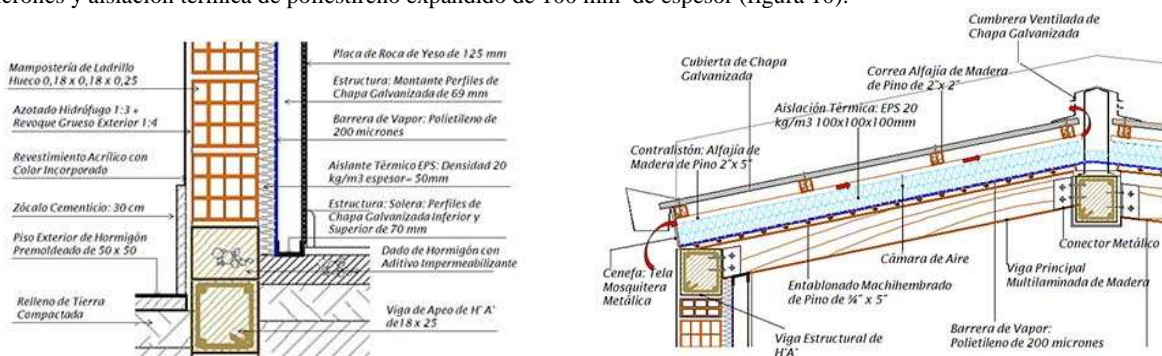
Figura 10: Características constructivas de muros y cubierta de la vivienda categoría 3 y 4
