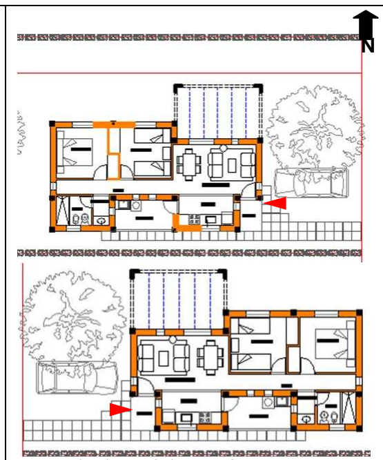
Figura 8: Plantas de la vivienda con acceso Este u Oeste
