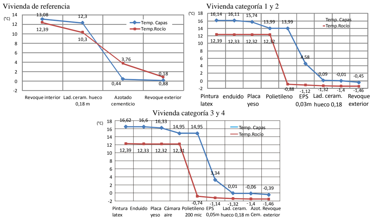
Figura 12: Verificación de riesgo de condensación intersticial en muros para las diferentes categorías de análisis.
