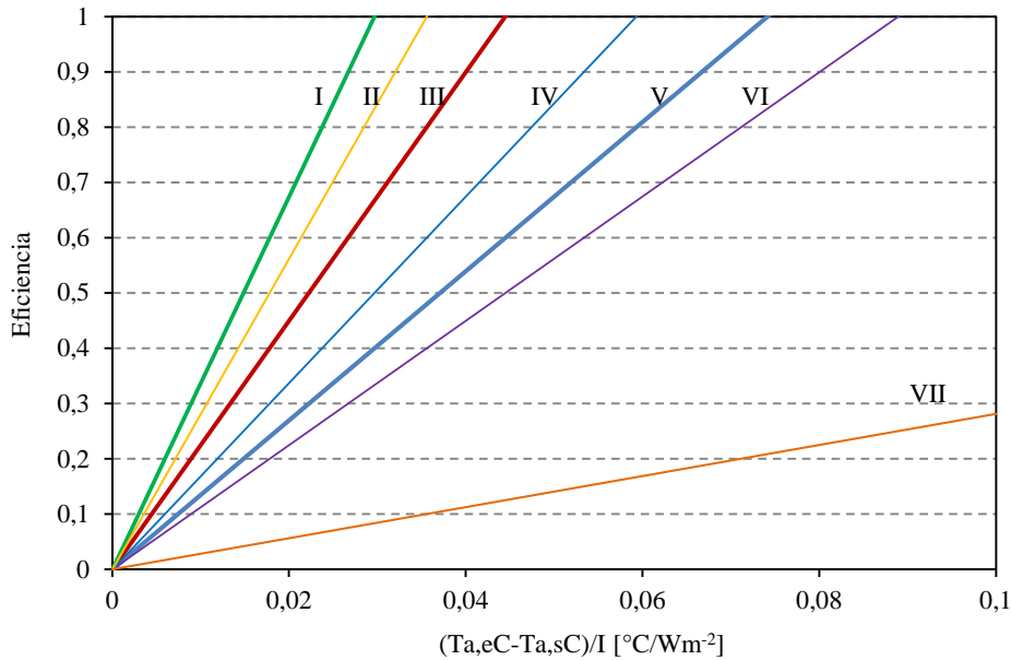
Figura 8. Eficiencia del colector en función de la relación \Delta T_a/I
