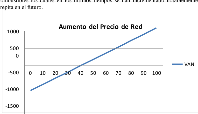
Figura 7: Variación del VAN ante el incremento del precio de red (Escenario 4)
