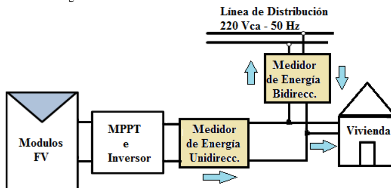
Figura 1: Sistema FV instalado en las Viviendas
