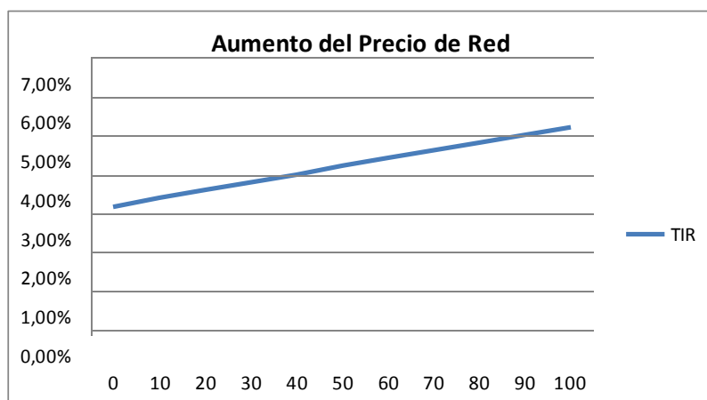
Figura 9: Variación de la TIR ante el incremento del precio de red (Escenario 4)
