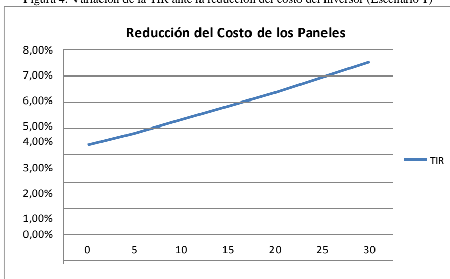
Figura 5: Variación de la TIR ante la reducción del costo de los paneles FV (Escenario 2)
