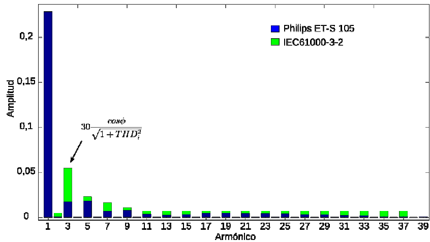
Figura 9: espectro de la corriente de entrada
