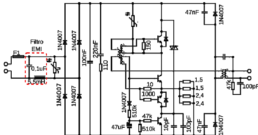
Figura 2: circuito esquemático
