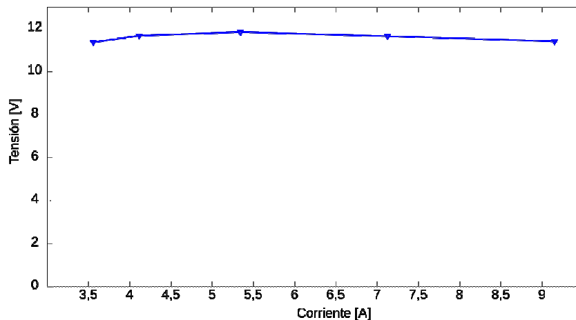
Figura 10: regulación de la salida
