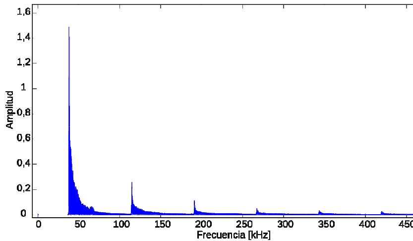
Figura 8: espectro de la corriente de salida
