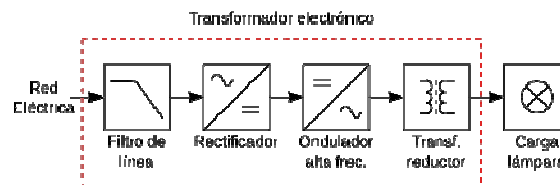
Figura 3: diagrama de bloques del transformador electrónico
