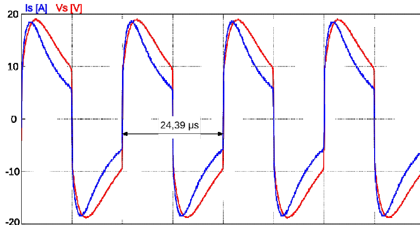
Figura 7: detalle de la corriente y tensión de salida
