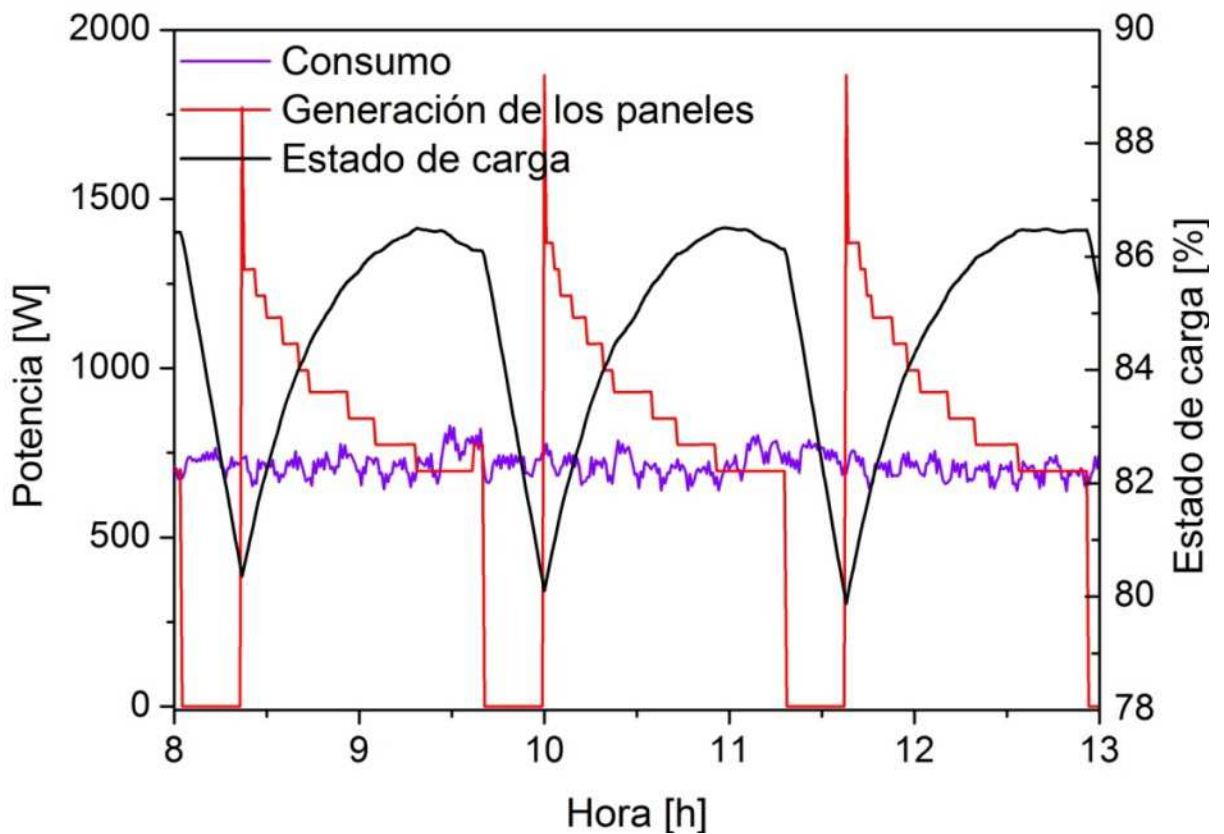
Figura 5: Consumo, potencia generada por el panel solar y estado de carga de la batería en la simulación realizada para día 30 de junio para el satélite SAC-D.
