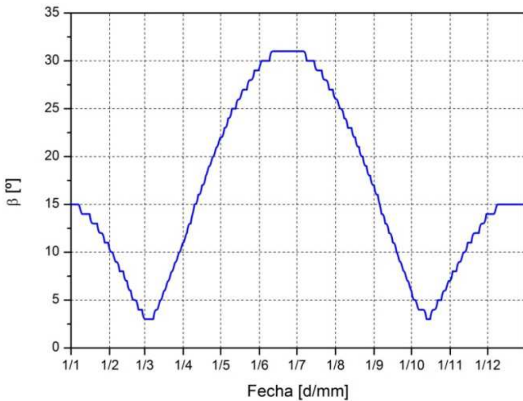
Figura 3: Perfil del ángulo de incidencia de la radiación solar sobre los paneles del satélite SAC-D.
