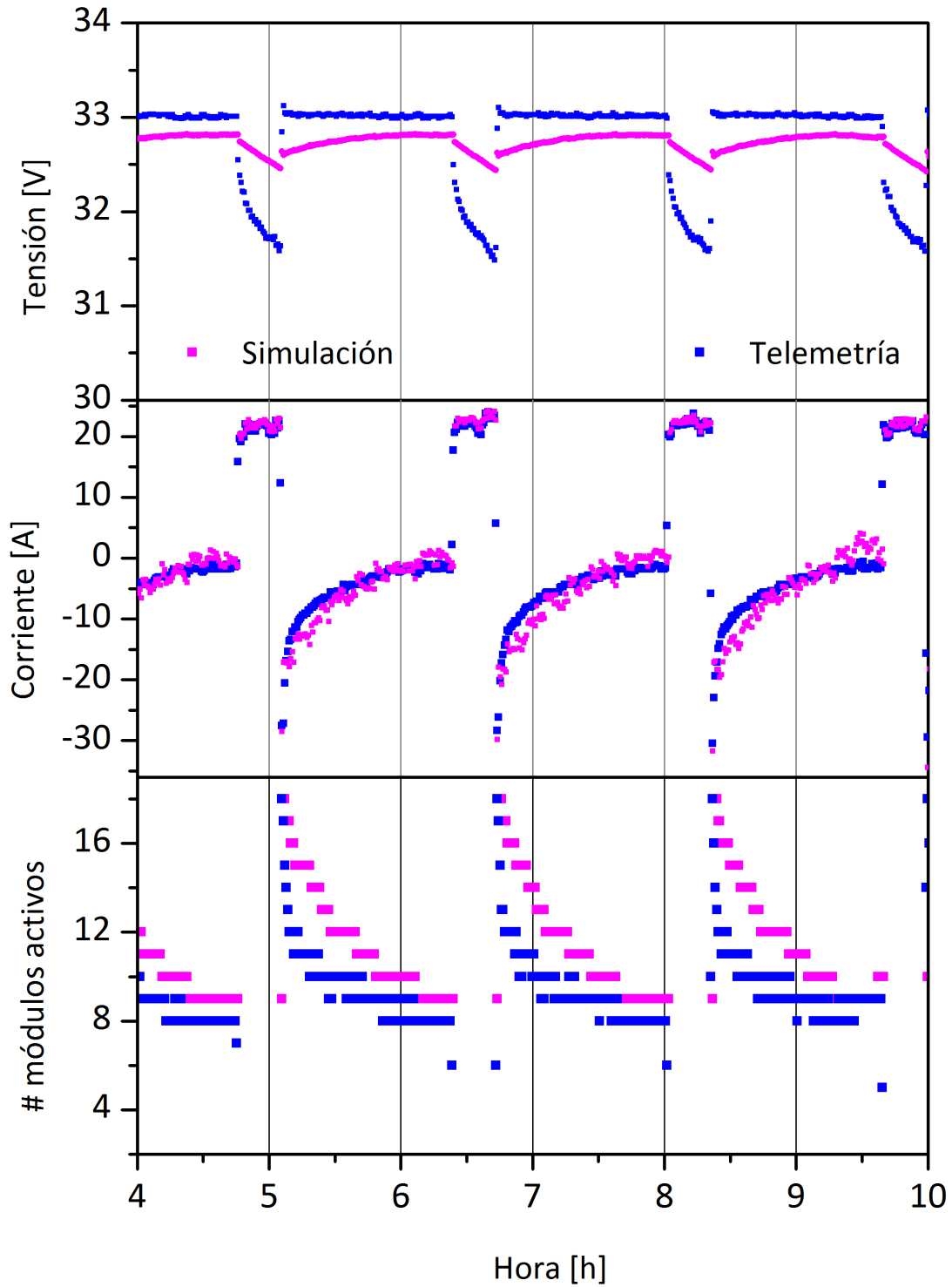
Figura 7: Comparación de los resultados de la simulación con los valores de la telemetría para el 20 de junio de 2013: tensión (arriba) y corriente (centro) en los bornes de la batería y cantidad de módulos activos (abajo) para el satélite SAC-D.
