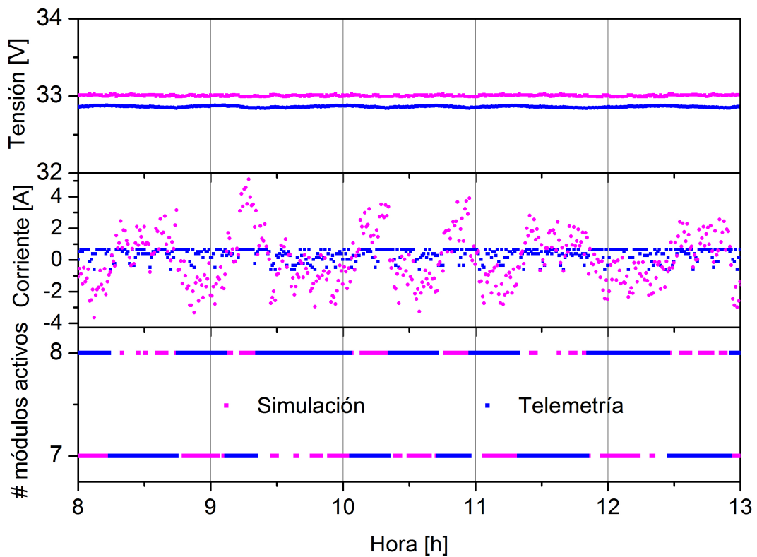
Figura 6: Comparación de los resultados de la simulación con los valores de la telemetría para el 30 de diciembre de 2012: tensión (arriba) y corriente (centro) en los bornes de la batería y cantidad de módulos activos (abajo) para el satélite SAC-D.
