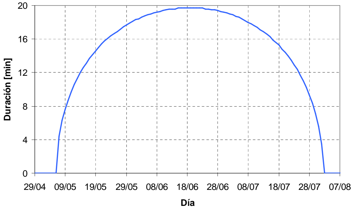
Figura 2: Perfil de duración del eclipse para el satélite SAC-D.
