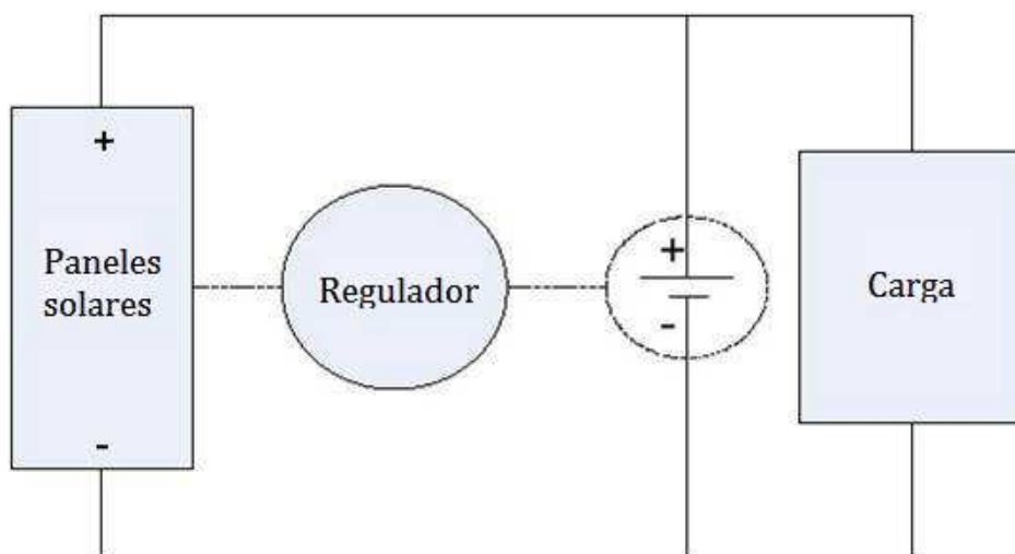
Figura 1: Esquema simplificado de un subsistema de potencia de un satélite.
