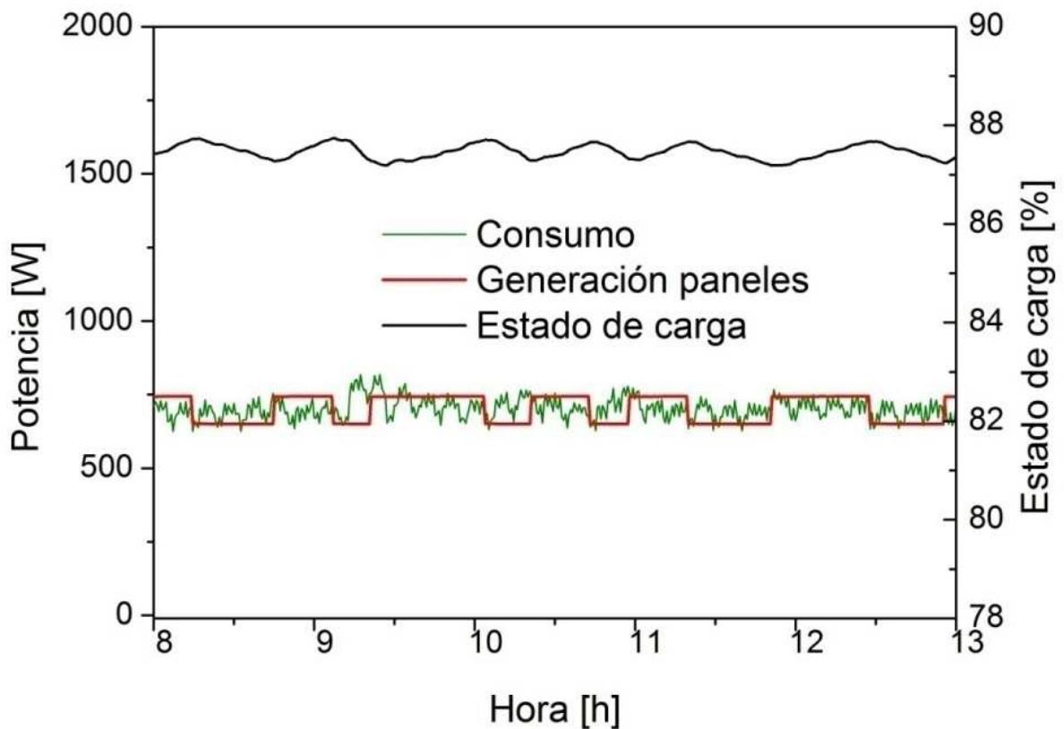
Figura 4: Consumo, potencia generada por el panel solar y estado de carga de la batería en la simulación realizada para día 30 de diciembre para el satélite SAC-D.
