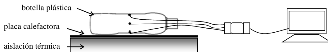
Figura 1: Esquema de la experiencia con la botella plástica rellena con viruta.
