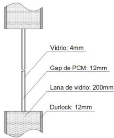
Figura 8. Configuración de ventana – pared frontal.
