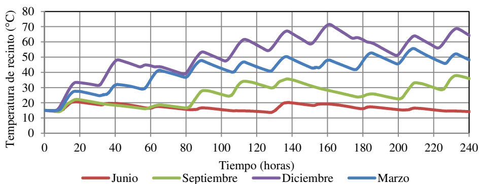
Figura 15. Temperatura interior del recinto.
