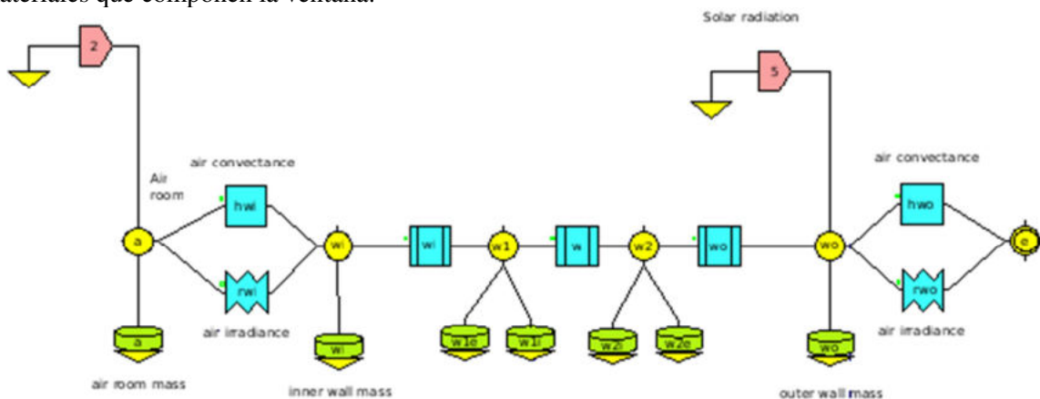
Figura 9. Circuito térmico de ventana con PCM.
