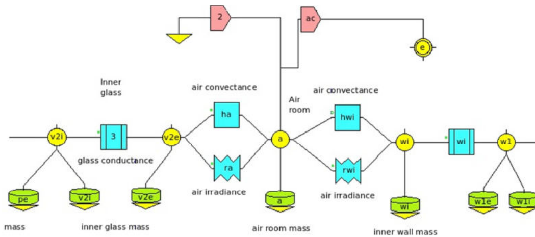
Figura 18. Sistema de control de temperatura mediante acondicionador de aire.
