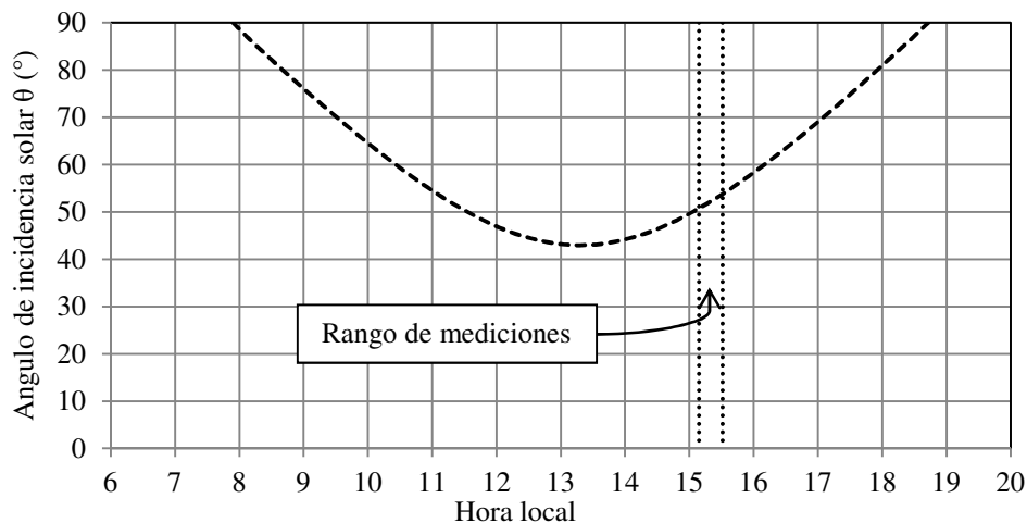
Figura 6. Variación del ángulo de incidencia para el día 12/05/2017.
