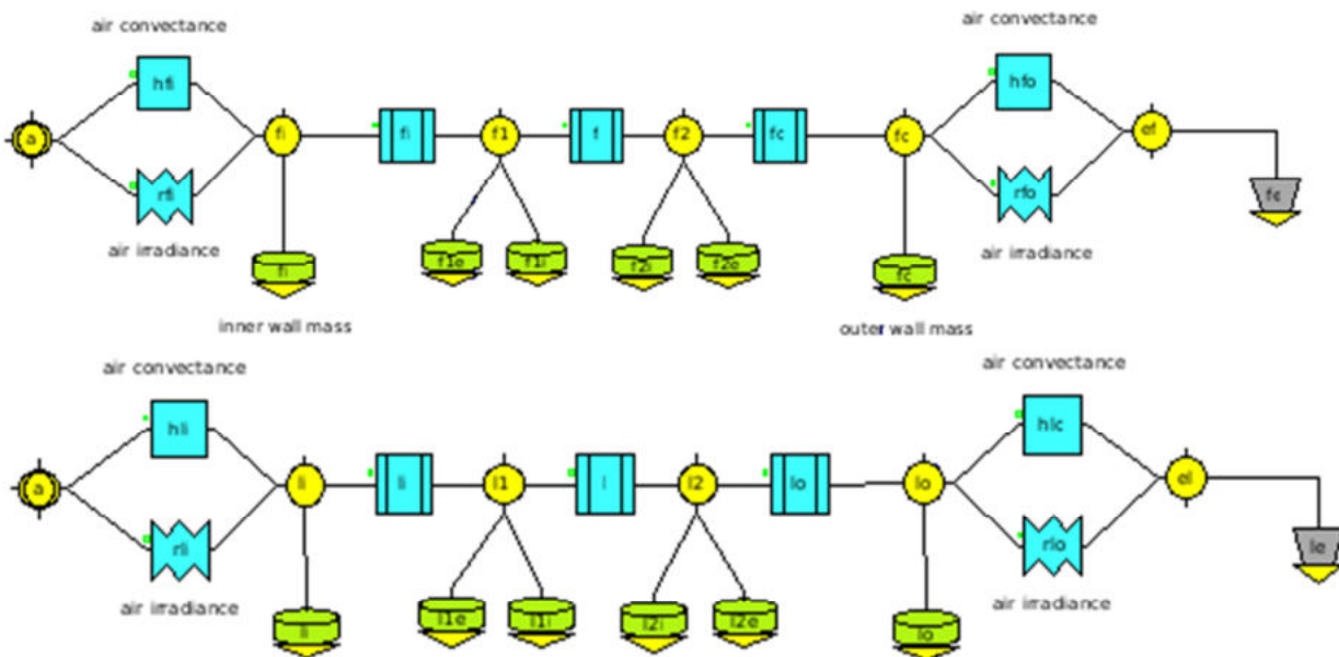
Figura 11. Circuitos térmicos para pared de fondo (arriba) y cerramientos laterales (abajo).
