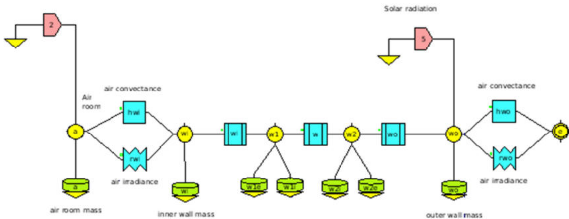
Figura 10. Circuito térmico de pared frontal, orientada hacia el norte.
