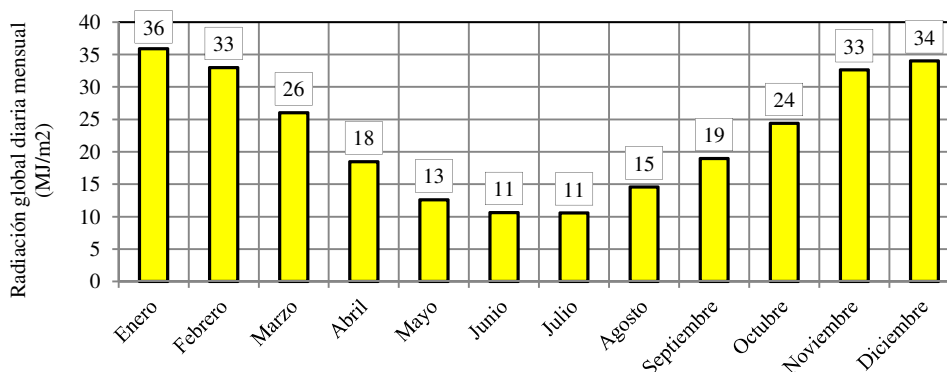
Figura 13. Radiación global horizontal promedio diario mensual para Santiago de Chile.
