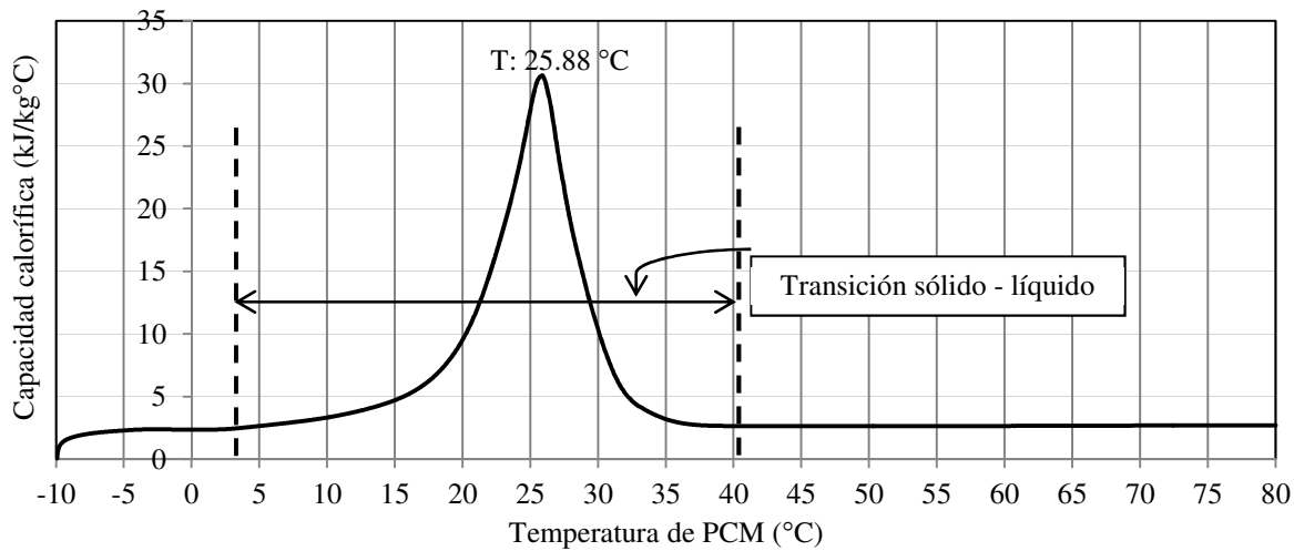
Figura 4. Curva representativa de la capacidad calorífica del PCM.
