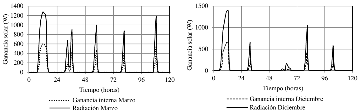
Figura 17. Curvas de ganancia solar en el interior de los recintos y potencia térmica incidente en ventana.
