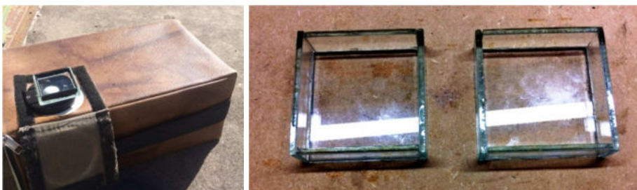
Figura 5. Izquierda: celda con PCM sobre instrumento Li-1800. Derecha: celdas vacías.
