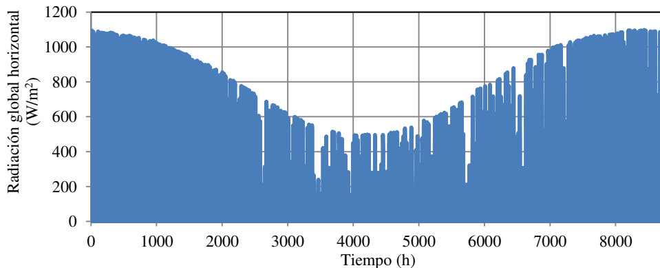
Figura 2: Radiación global sobre plano horizontal medida en Santiago de Chile.
