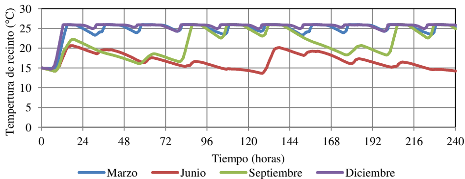
Figura 19. Temperaturas del recinto con limitación por aire acondicionado.
