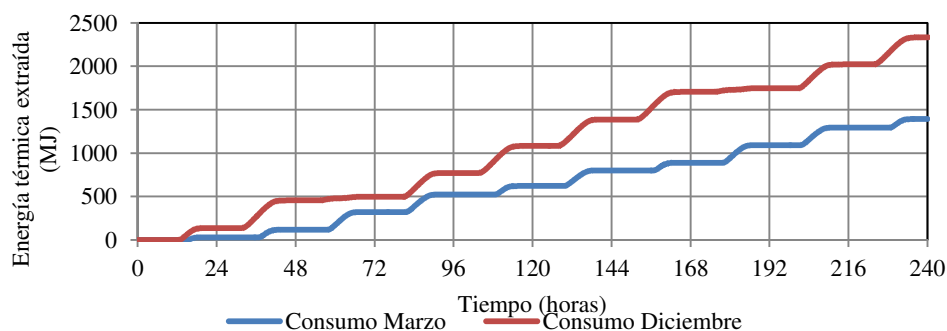
Figura 20. Energía térmica a extraer del recinto para control de temperatura.
