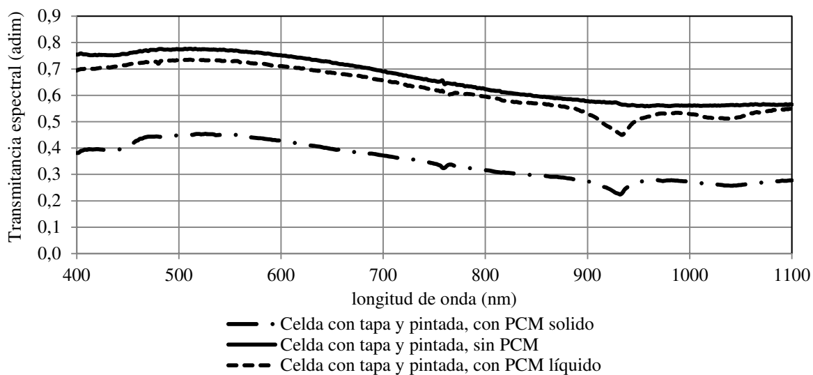
Figura 7. Transmitancia espectral de las muestras.
