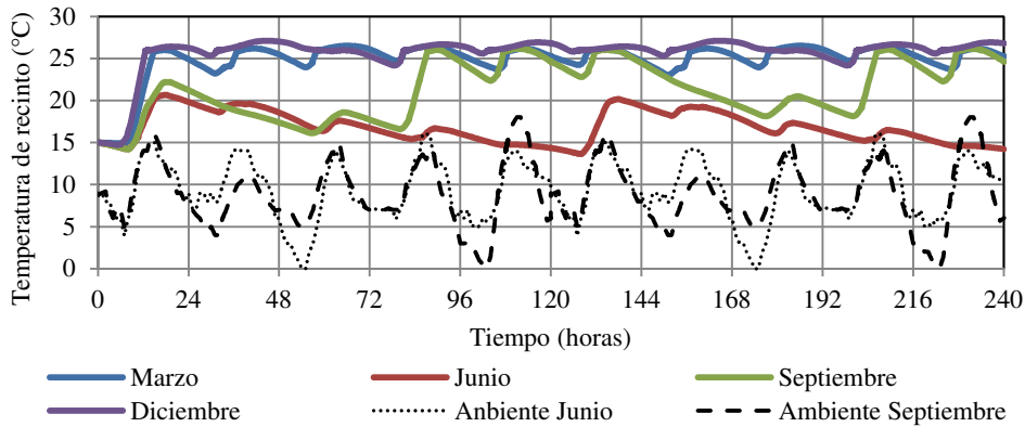
Figura 16. Temperatura de recinto con estrategia de sombreado.
