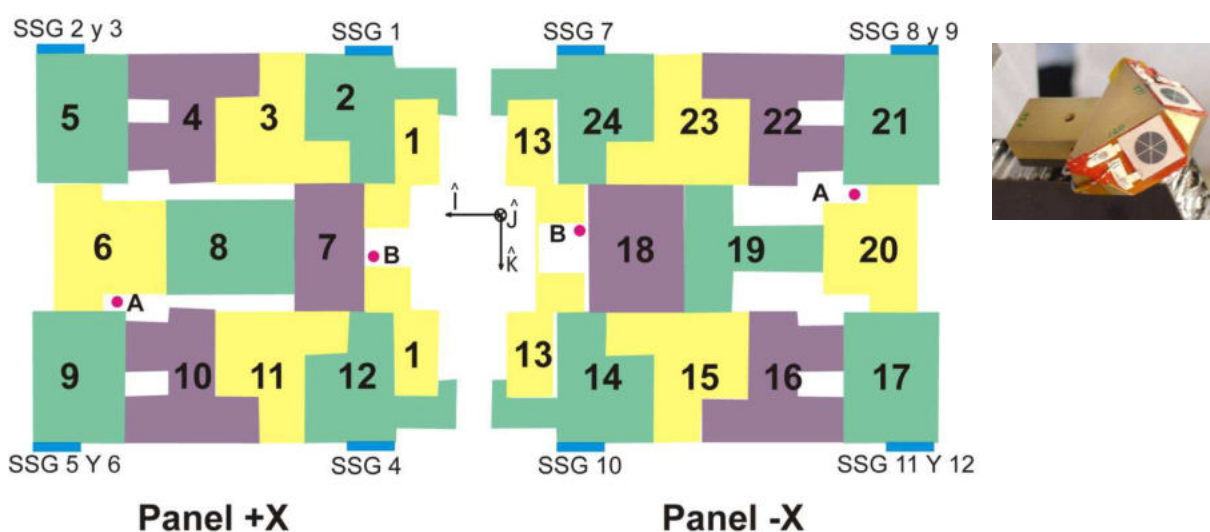
Figura 1: Conformación de los paneles solares del satélite SAC-D y SSG 8 y 9 sobre su soporte. Los rectángulos celestes indican la posición de los sensores solares gruesos y los puntos rojos, la de los sensores de temperatura.
