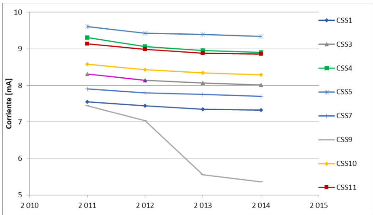
Figura 4: Valores de los promedios de las corrientes de los SSG 1, 3 4, 5, 7, 9, 10 y 11 durante la misión
