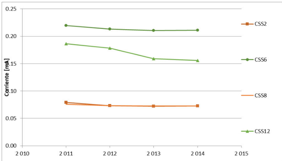
Figura 3: Valores de los promedios de las corrientes de los SSG 2, 6, 8 y 12 durante la misión
