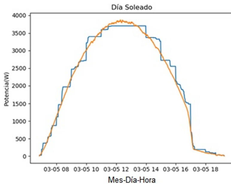
Figura 5. Potencia generada y predicción para un día soleado.
