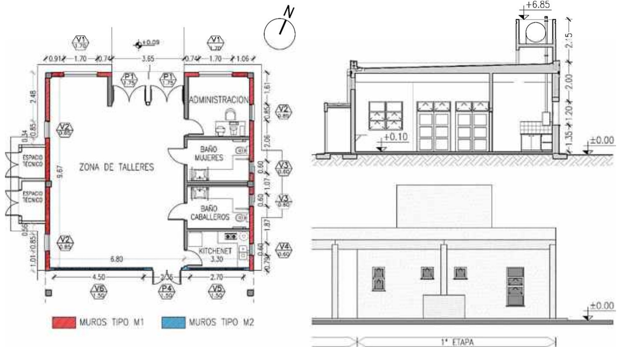
Fig. 2: Planta, corte y fachada del proyecto del edificio.
