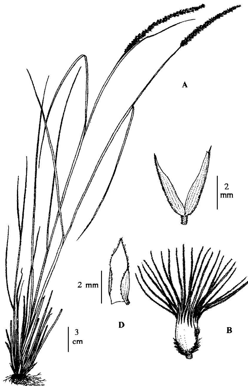
Lám. 4. Pappophorum vaginatum . A, planta; B, espiguilla sin glumas; C, glumas; D, pálea. (De Novara, 4559). Dib. M. C. Otero.
