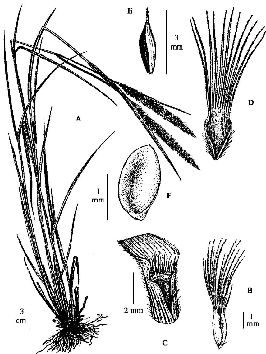
Lám. 3. Pappophorum pappiferum . A, planta; B, espiguilla sin glumas; C, cuello de la vaina; D, fruto. (De Novara, 3083). Dib. M. C. Otero.
