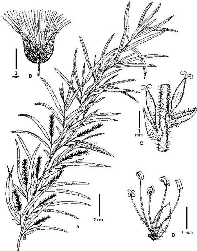
Lám. 1. Salix humboldtiana . A, rama; B, fruto luego de la dehiscencia; C, fracción de amento con 2 flores pistiladas; D, flor estaminada; (A y C, de Núñez 300; B, de Tolaba 276; D, de Novara 5635B). Dib. L. J. Novara
